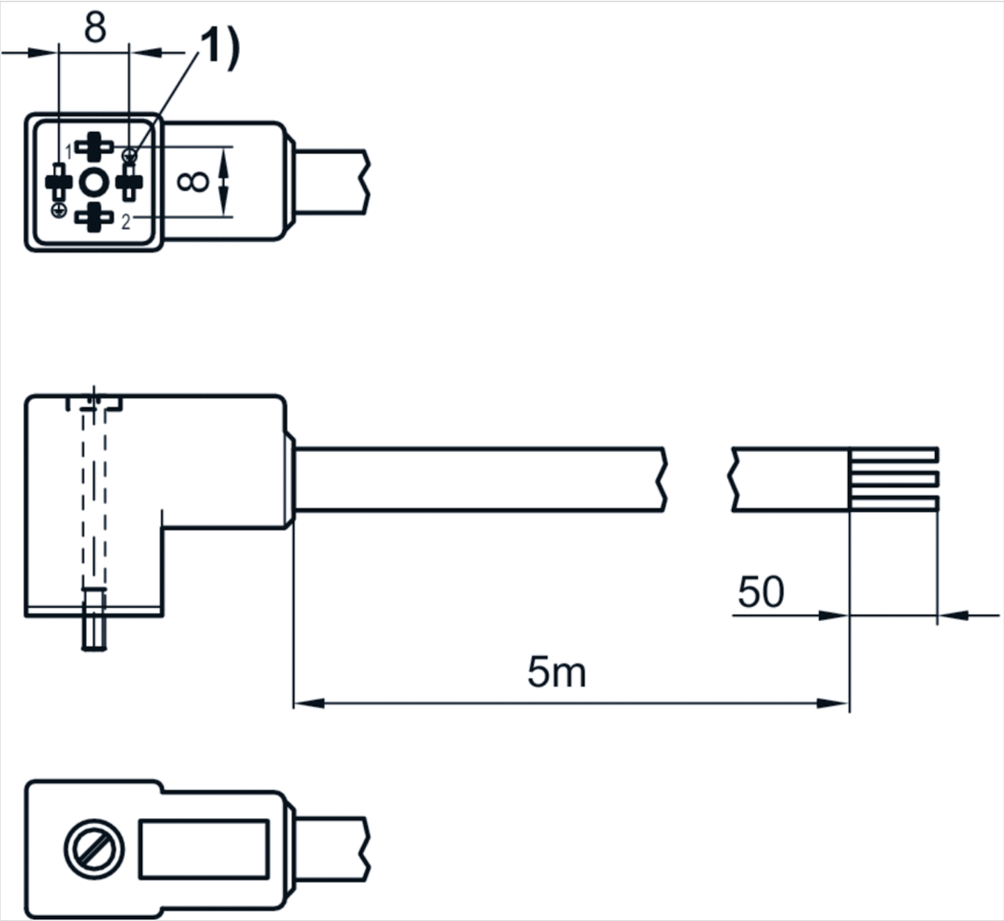
1) Coding pin
